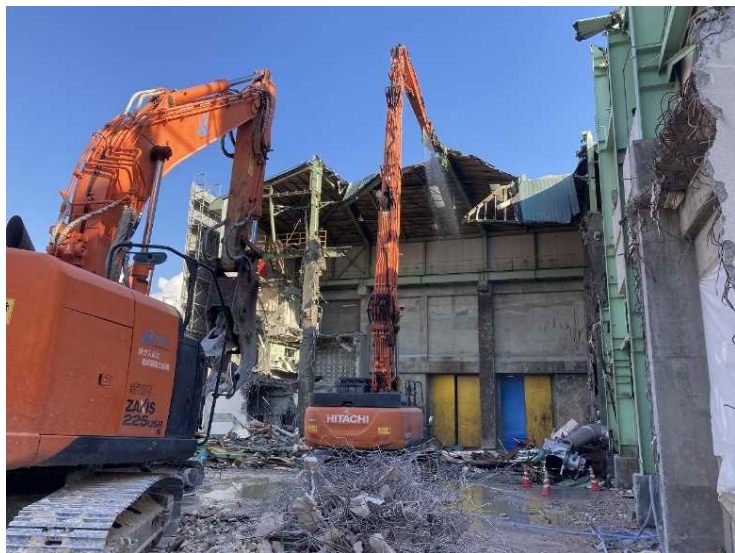
⑤ 工場棟 建屋屋根解体状況
