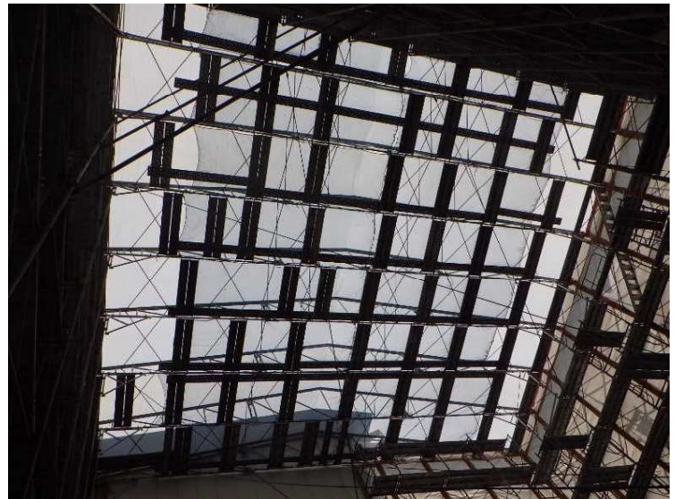
⑭ 工場棟 解体ヤード 前室屋根養生検査
