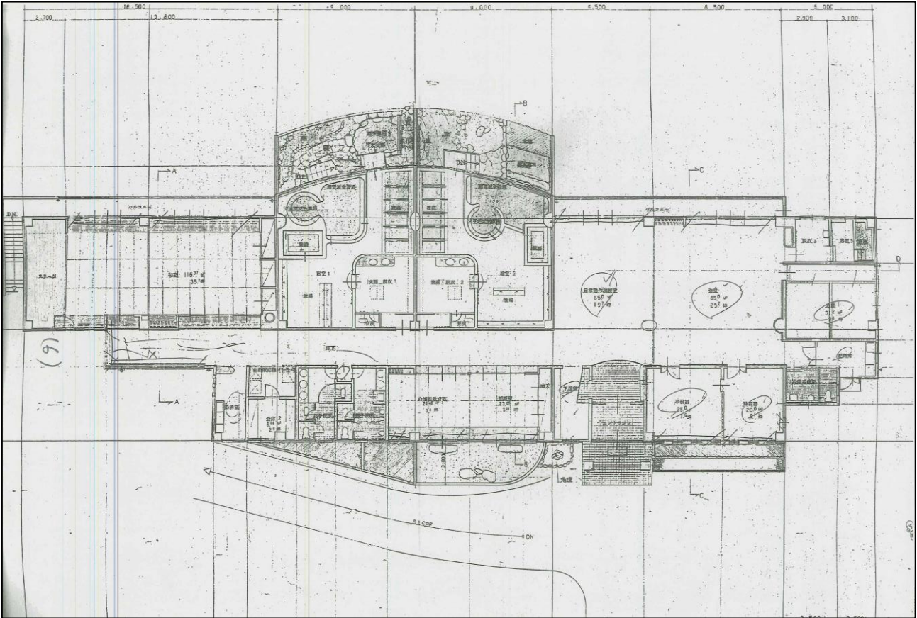
平面图（2F）
