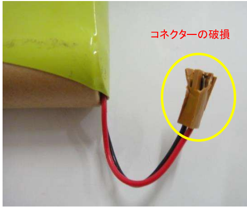
(コネクタ一部の破損) コネクタ内でリード線同士が接触し 短絡の可能性あり
